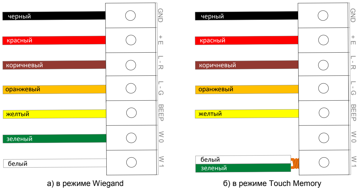
Рисунок 7. Подключение считывателя
