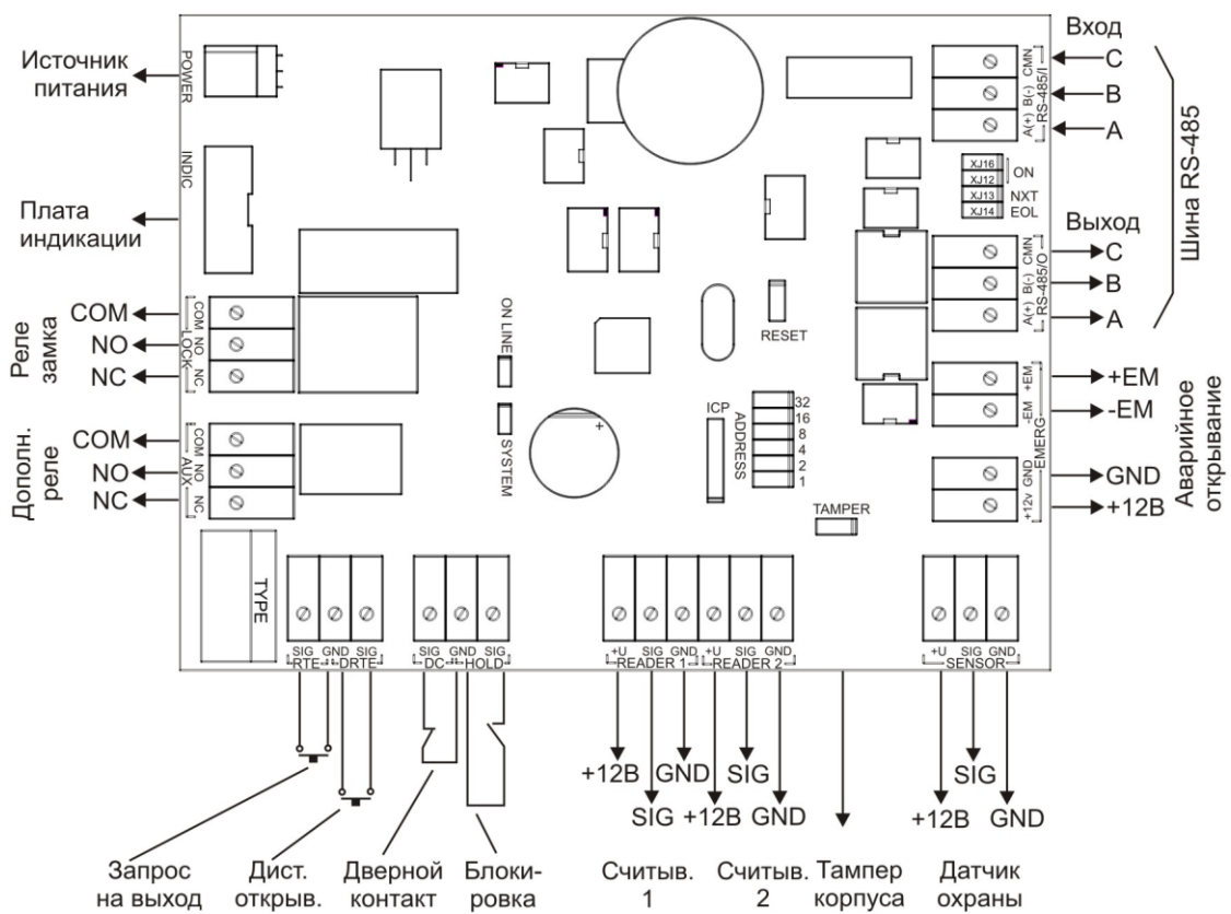
Рисунок 3. Схема платы контроллеров NC-1000M/NC-5000
