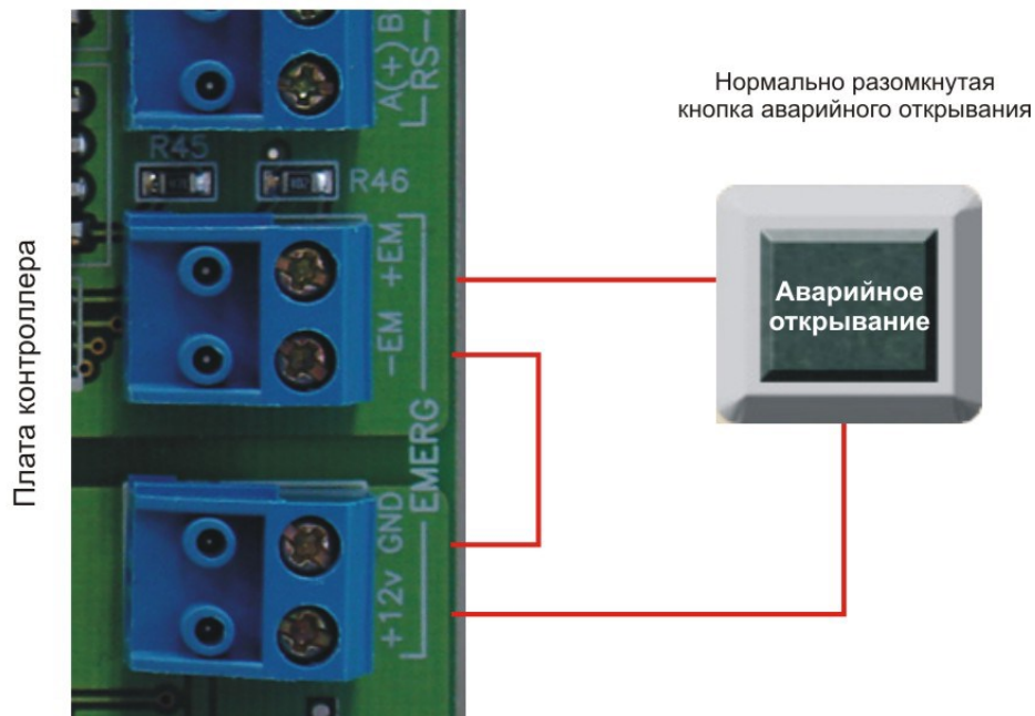
Рисунок 22. Подключение кнопки аварийного выхода к одному контроллеру
