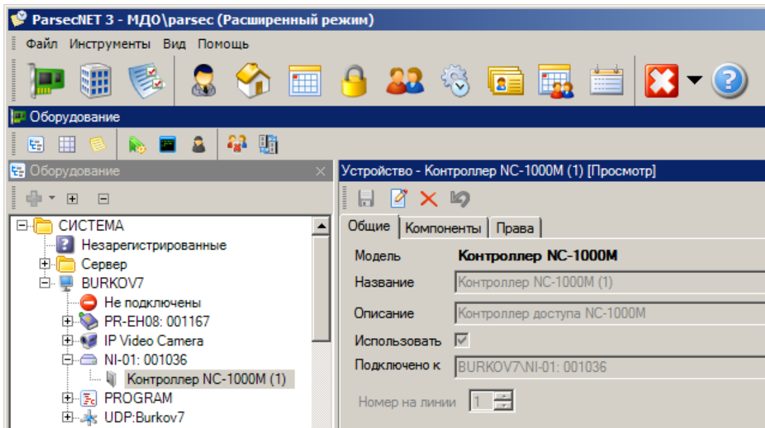
Рисунок 29. Настройка контроллера в ParsecNET 3
