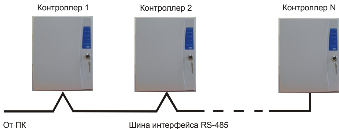
Рисунок 26. Соединение контроллеров по топологии «Шина»
