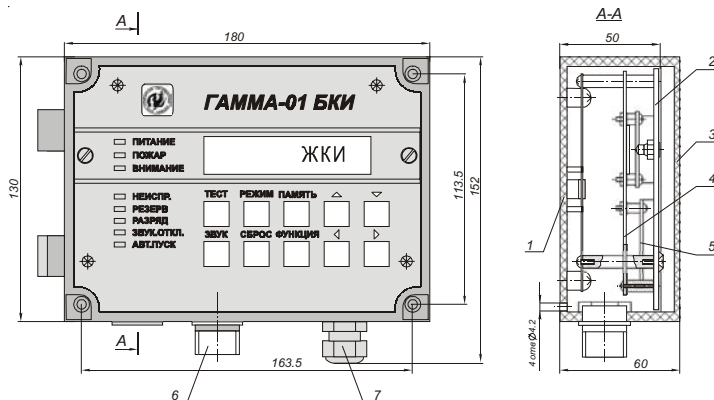
Блок клавиатуры и индикации «Гамма-01 БКИ»: 1 - корпус; 2 - панель; 3 - крышка; 4 - плата; 5 - плата; 6 - вилка 2PM22B10Ш1В1; 7 - гермоввод.
