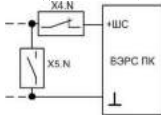
Рис.7. Схема включения охранных извещателей в ШСО.
