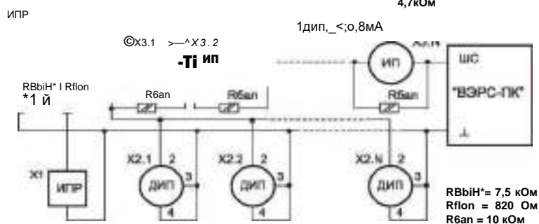
Рис.5. Комбинированная схема включения ШС. Однопороговый алгоритм с верификацией.
