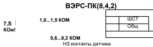
Рис.8. Схема включения технологических датчиков в ШСТ.
