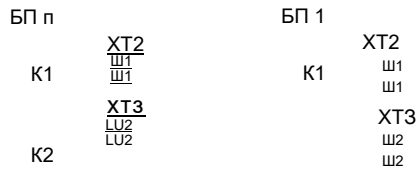
Рис.6. Схема включения линейных дымовых извещателей ИПДЛ-Д-П/4Р.
